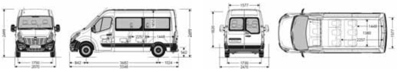
Combi L2H2
